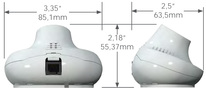
Rückansicht
